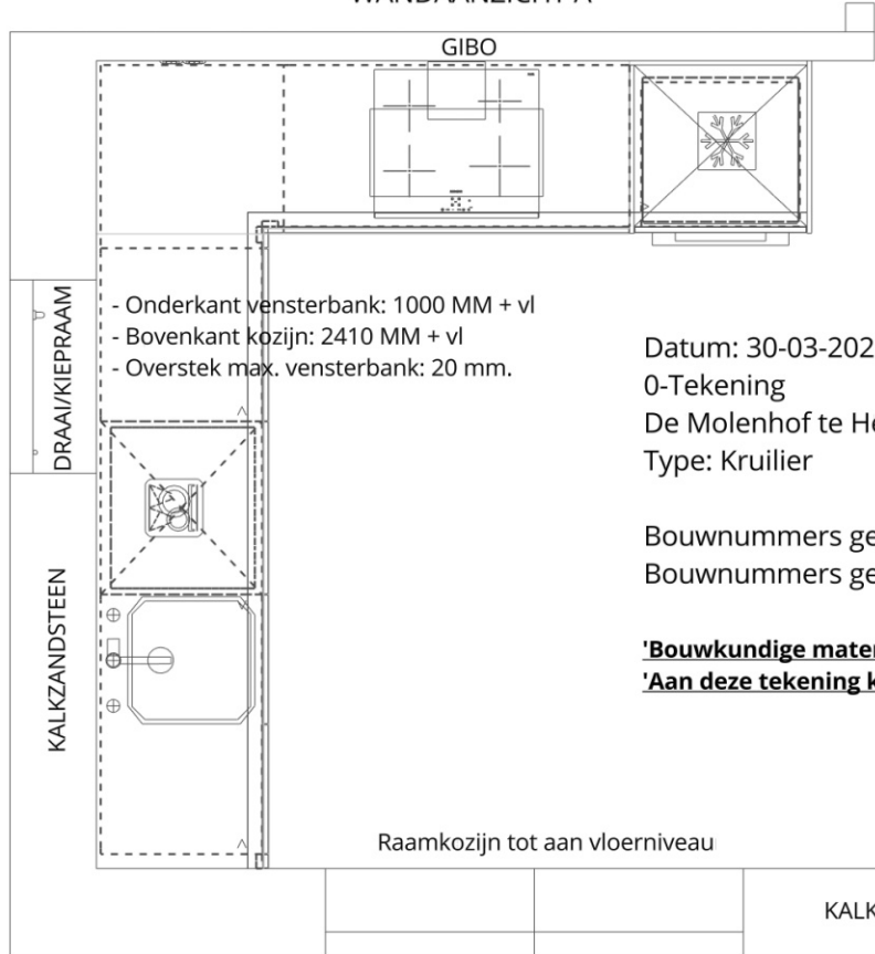
WANDAANZICHT A
